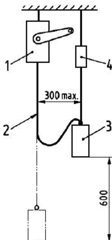
Рисунок 1 - Методика проверки динамической рабочей характеристики для спасательного подъемного устройства класса В
